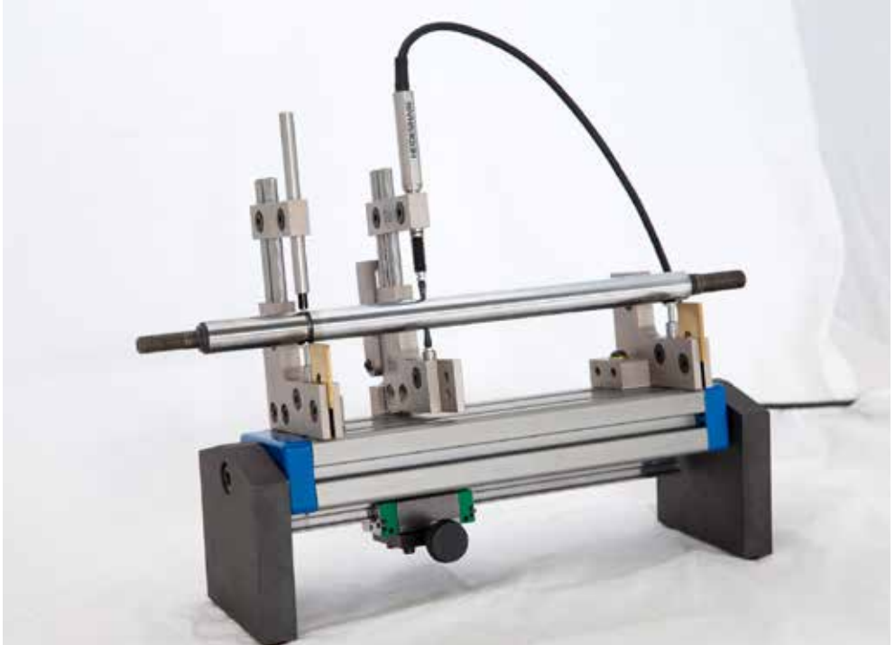
Lineareinheit zum Prüfen von Geradheit und Zylindrizität
