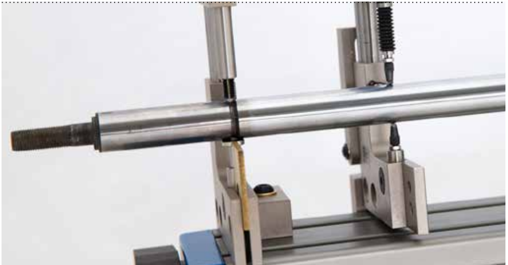
Lineareinheit zum Prüfen von Geradheit und Zylindrizität
